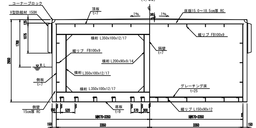
基本寸法図
